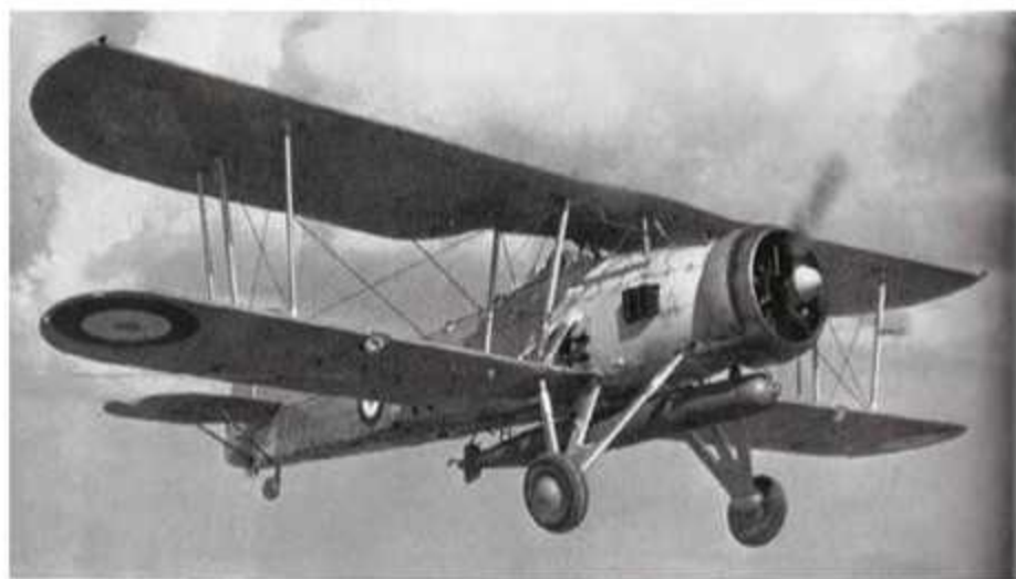
Biplano bombardero-torpedero Fairey Swordfish, avión poco potente y desfasado en 1940, pero que en Tarento hizo valer su robustez y la destreza de sus pilotos para convertirse en el arma fundamental que desventró los acorazados italianos en su base.
